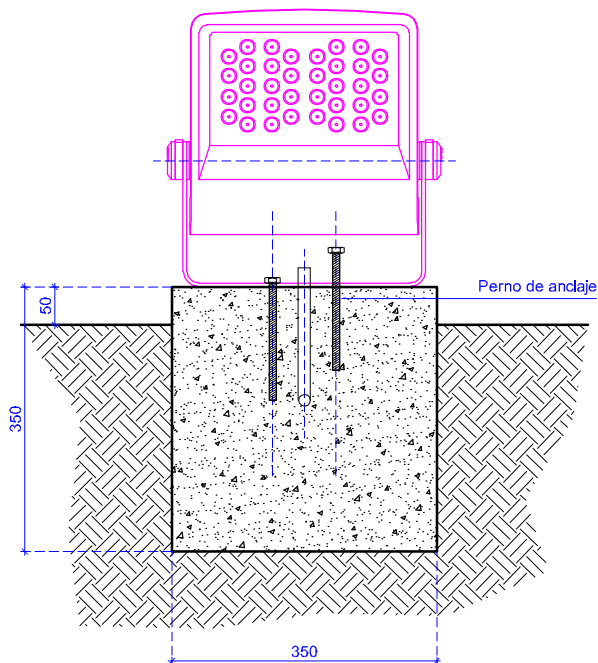
DETALLE DE ANCLAJE VISTA FRONTAL esc. 1:10
