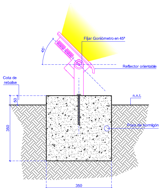
DETALLE DE ANCLAJE VISTA LATERAL / POSICION VALIDA esc. 1:10
