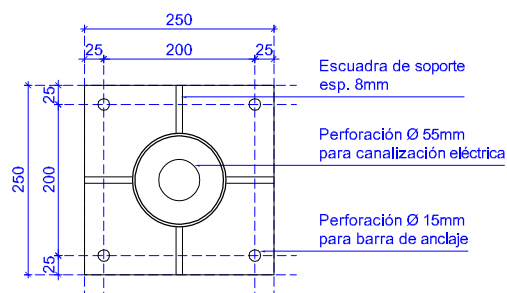
PLACA BASE DE ANCLAJE (Poste) esc. 1:10
