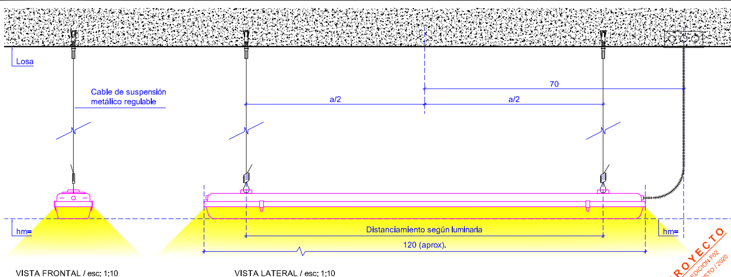
R03 ESQUEMA DE REFERENCIA / Luminaria hermética individual. / Colgante desde losa. / Bodegas y Sala eléctrica
