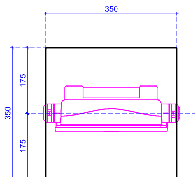
DETALLE DE ANCLAJE VISTA SUPERIOR esc. 1:10
