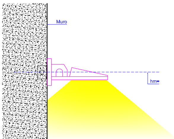
SECCION LATERAL / esc: 1:10
