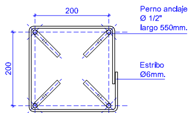
CANASTILLO DE ANCLAJE esc. 1:10
