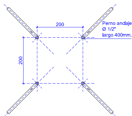
PERNOS DE ANCLAJE POSTE (EN LOSA) esc. 1:10
