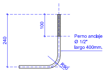
PERNO DE ANCLAJE esc. 1:10
