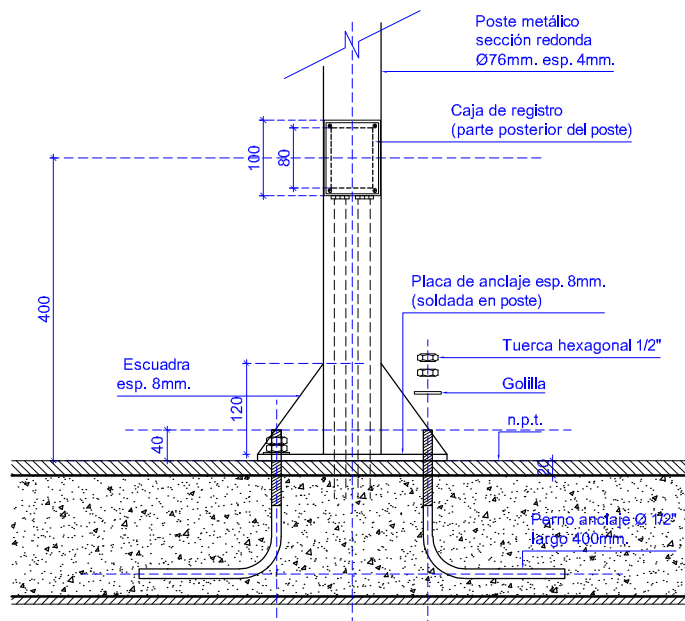
DETALLE ANCLAJE POSTE (EN LOSA) esc. 1:10
