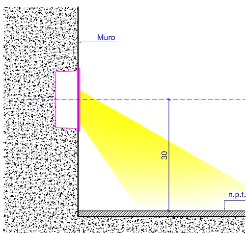
SECCION LATERAL / esc: 1:10
