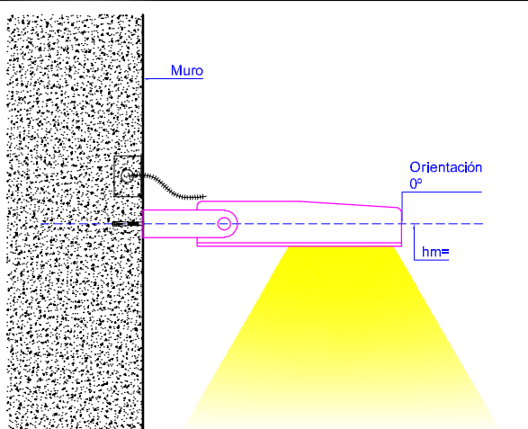
SECCION LATERAL / esc: 1:10
