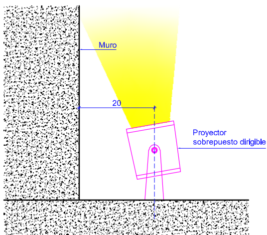
SECCION LATERAL / esc: 1:10
