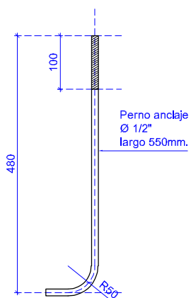
PERNO DE ANCLAJE esc. 1:10
