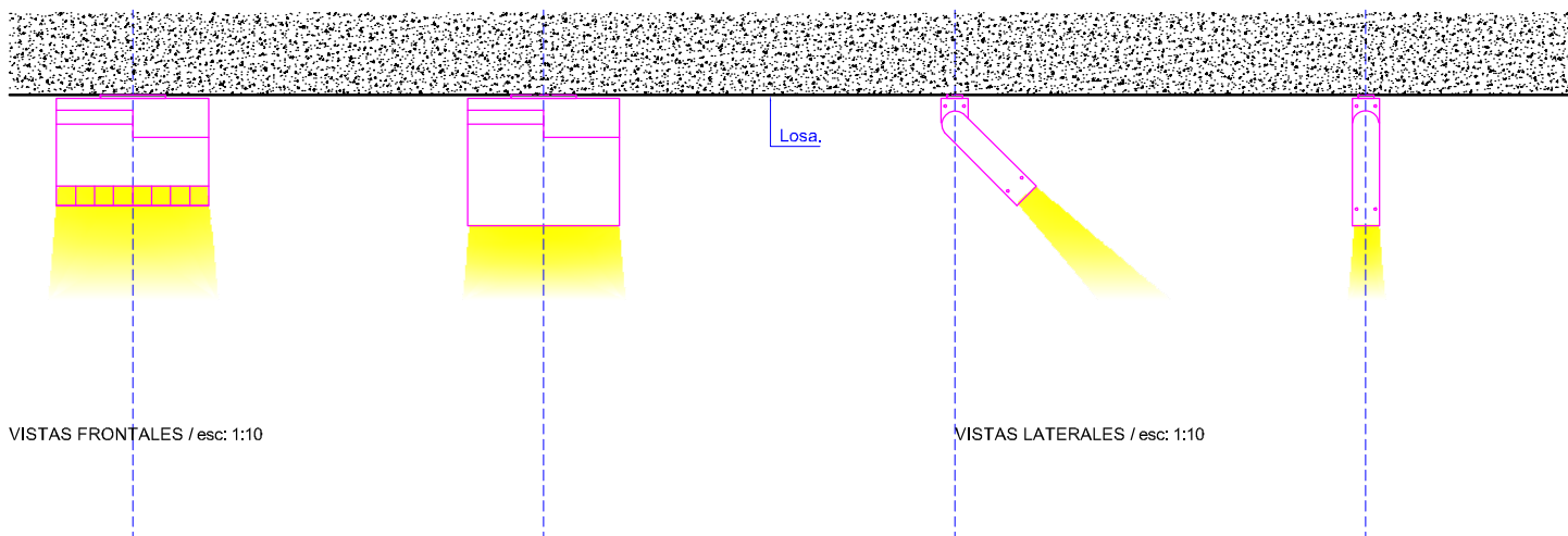
R13 ESQUEMA DE REFERENCIA / Luminaria tipo spot. / Sobrepuesta en losa o cielo. / Cripta.
