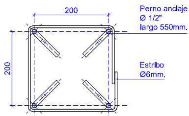
CANASTILLO DE ANCLAJE esc. 1:10
