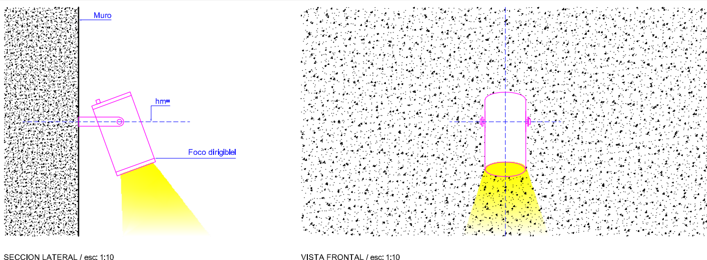
R02 ESQUEMA DE REFERENCIA / Luminaria tipo spot. / Adosada a muro o pilar. / Nave central y laterales.
