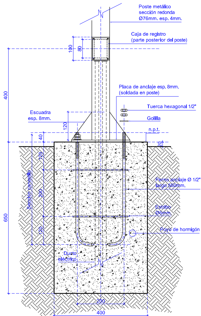
DETALLE ANCLAJE POSTE esc. 1:10
